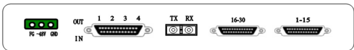
图 2. 设备后面板图
