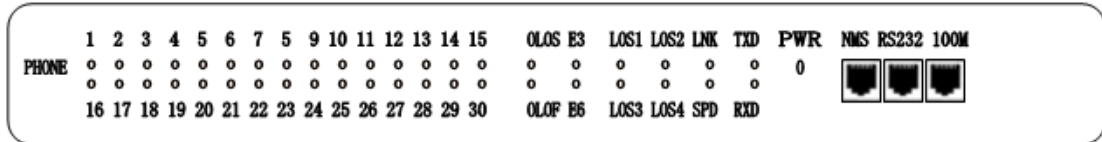
图 1. 复用设备前面板图
